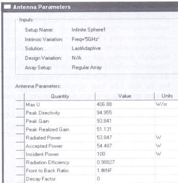
Fig. 3 Antenna parameters
