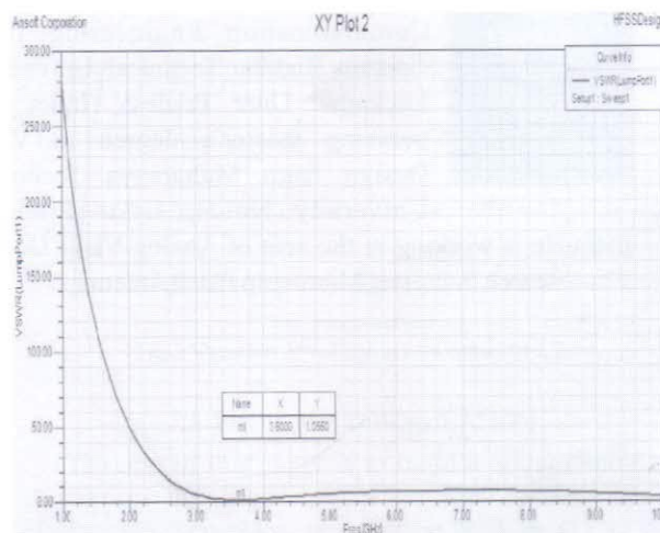
Fig. 5 VSWR
